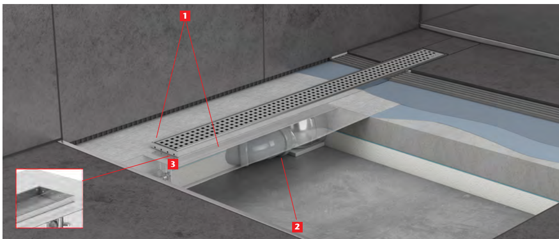
1. Prirubnica 2. Bočni izlivni priključak 3. Procedni otvori
