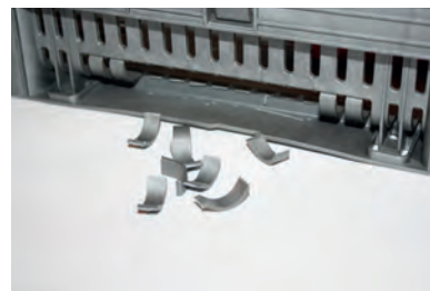
Rebra gurnuti ka spolja da dođe do loma.
