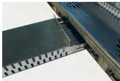
Vezni kanal, visine 5cm preklopiti na perforaciji.
