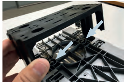
Postavite opruge u ležišta, i pritisnite element tako da upadne u odgovarajuće držače.
